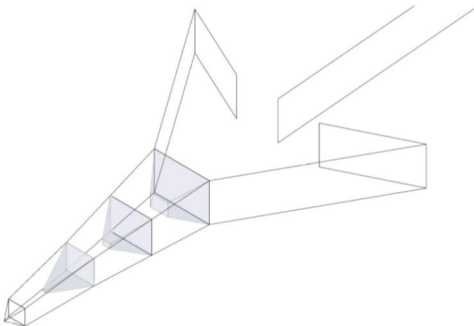
Joonis 2. Ühe kariaiaga ja eelkastita mõrd, kood 1KA0EK Allikas: Toomas Vikerpuur.
